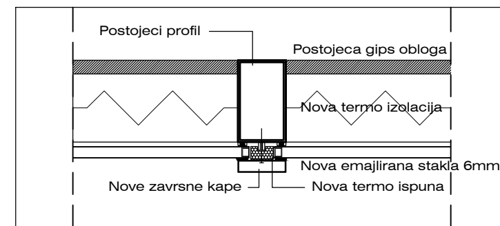
DETALJ NOVE FASADNE STOLARIJE
