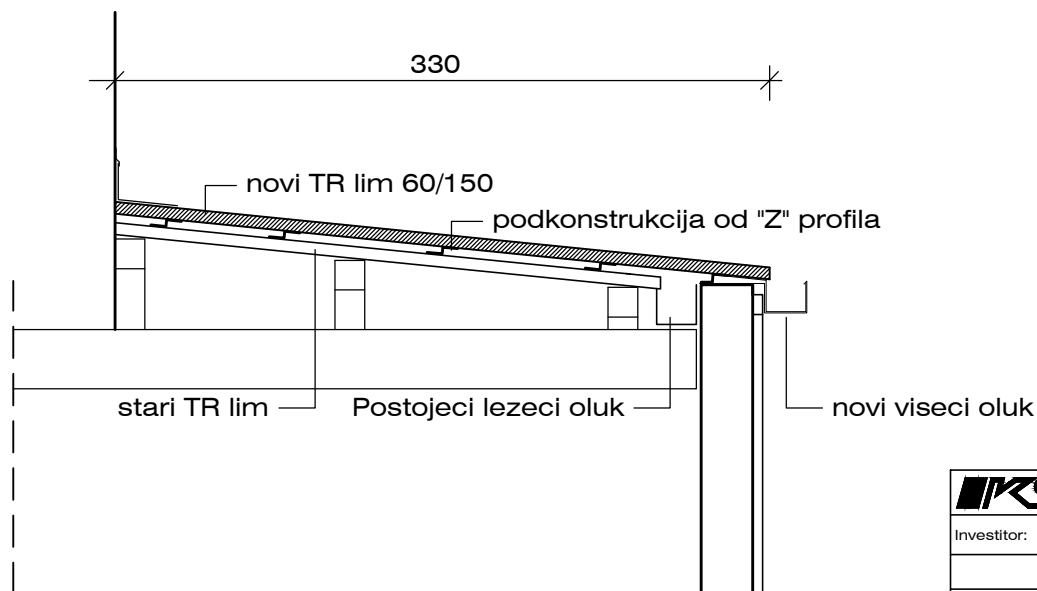
DETALJ POKRIVANJA KROVA NOVIM LIMOM R=1:25
