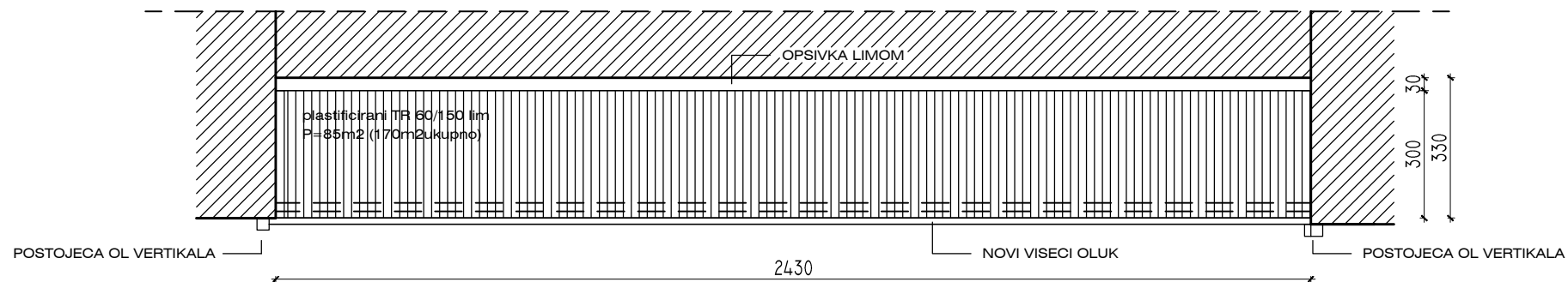
OSNOVA KROVA LEVE FASADE
