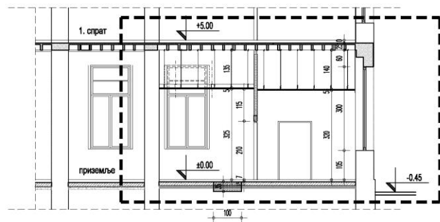
ПРЕСЕК 1-1
