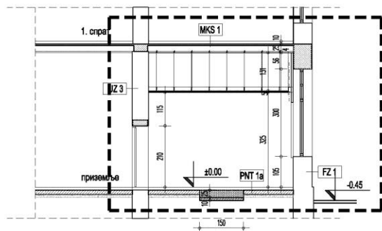
ПРЕСЕК 2-2
