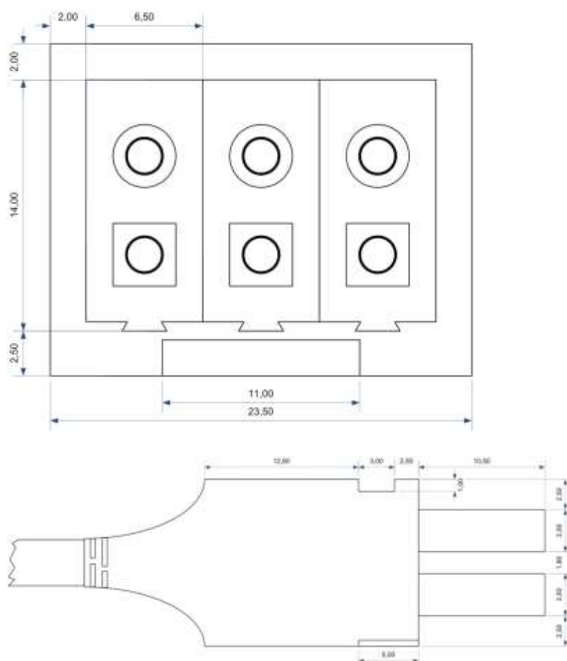
Слика бр. 2 – Трожилни ЕКГ кабл (lead wire) универзални
