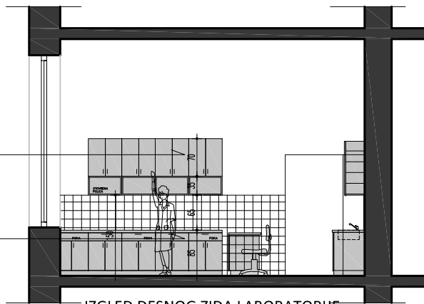
IZGLED DESNOG ZIDA LABORATORIJE
